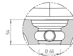
C 1:4
